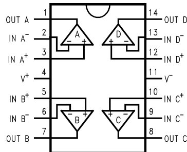
引脚功能
