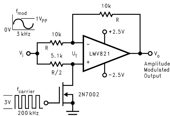
图 40. 调幅器电路
