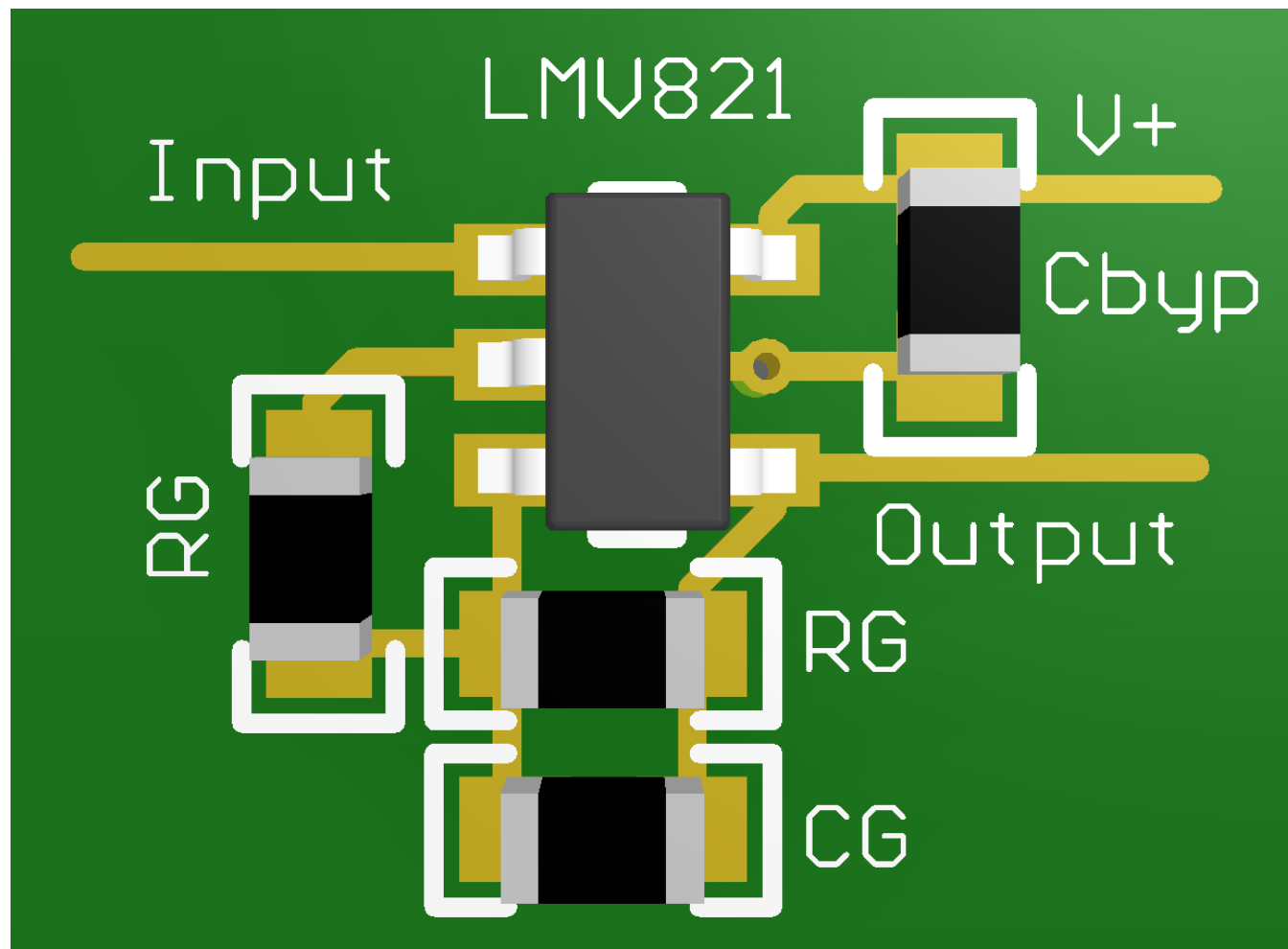
图 48. 3D 布局
