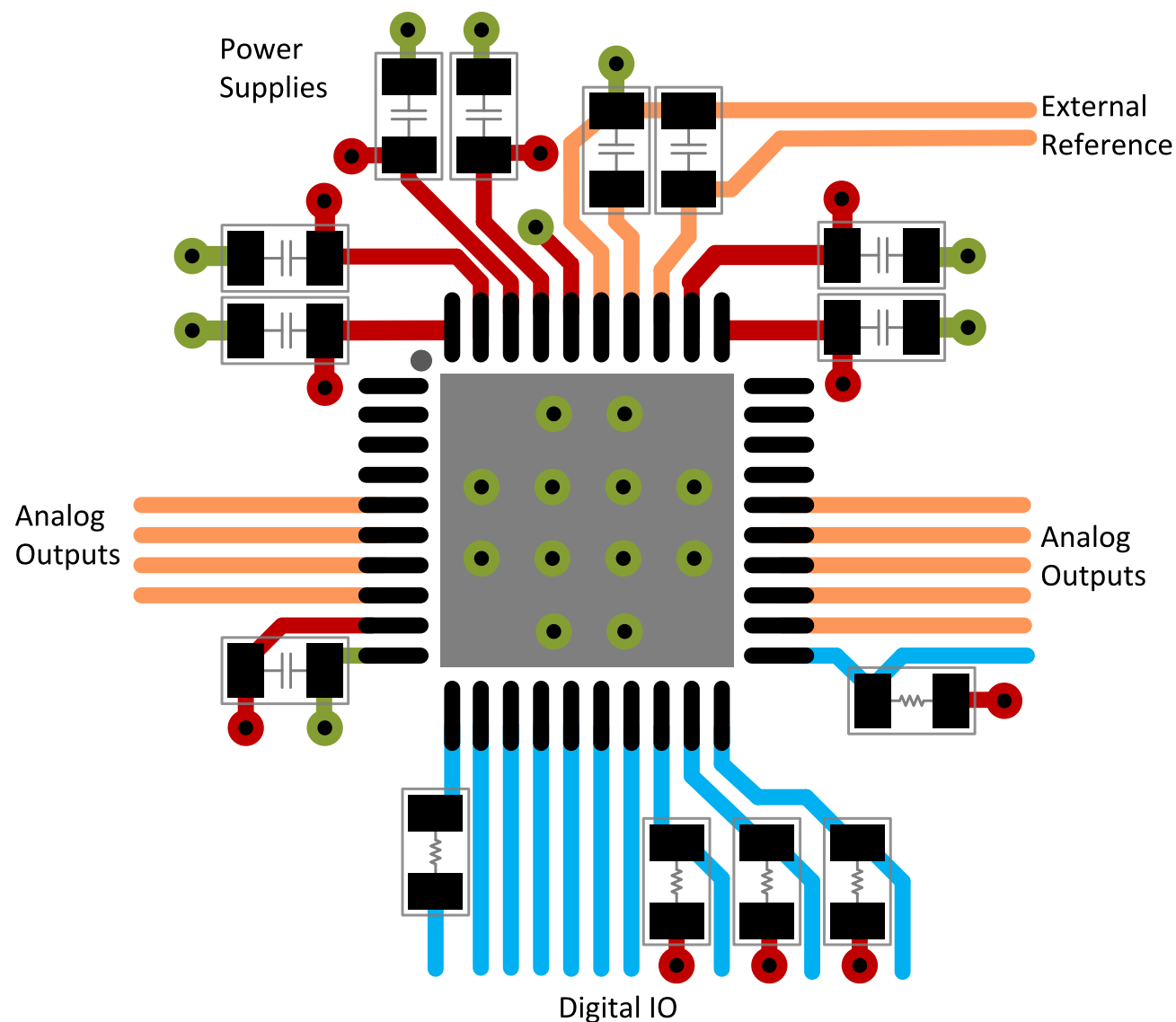
图 70. Example Layout
