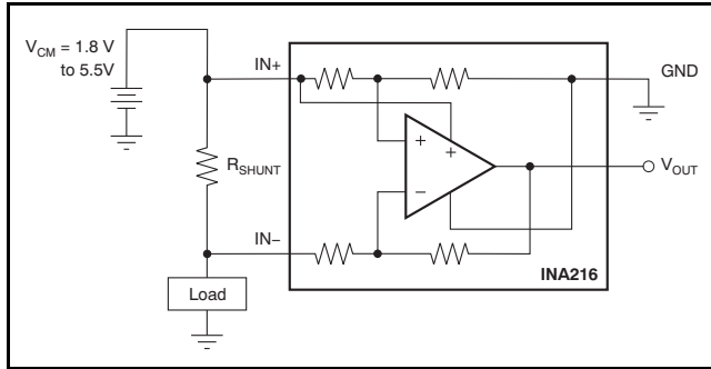
Figure 18. 典型应用
