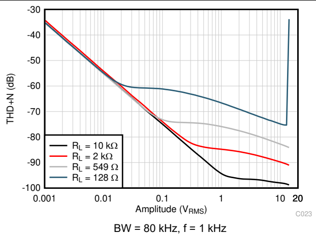
图 6-24. THD+N vs Output Amplitude
