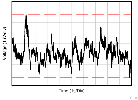
图 6-21. 0.1-Hz to 10-Hz Noise
