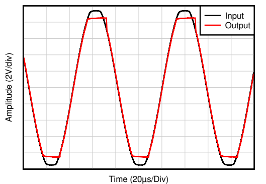
图 7-9. No Phase Reversal
