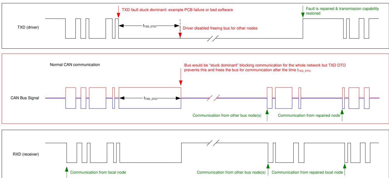
图 10-4. Timing Diagram for TXD DTO
