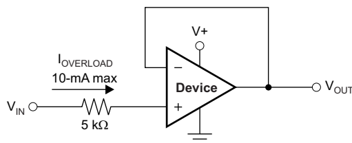
图 31. 输入电流保护
