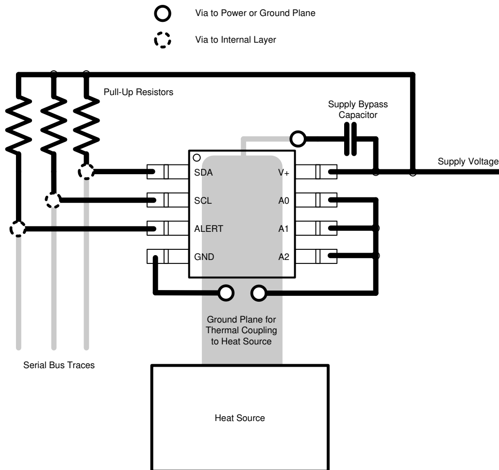
图 10-1. Layout Example
