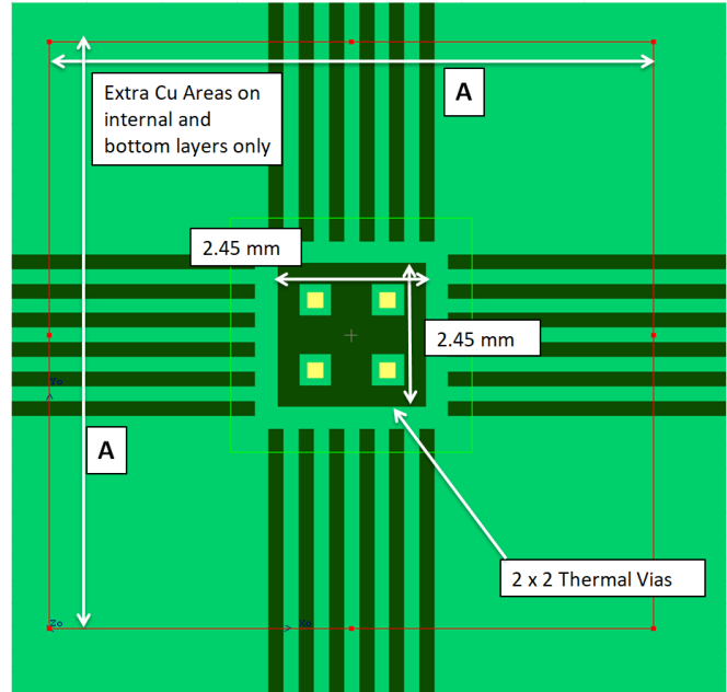
图 63. PCB - Top Layer (4/2-Layer PCB) for VQFN Package
