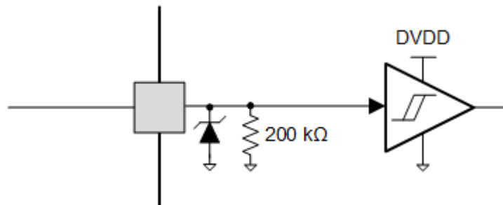
图 26. Logic-Level Input Pin Diagram
