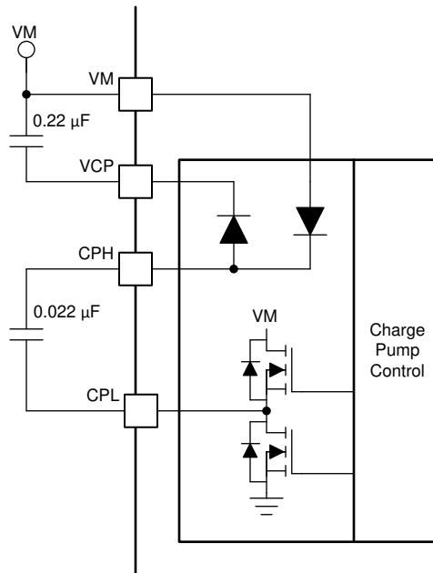
图 24. Charge Pump Block Diagram
