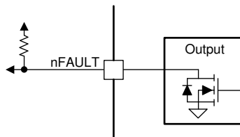
图 28. nFAULT Pin
