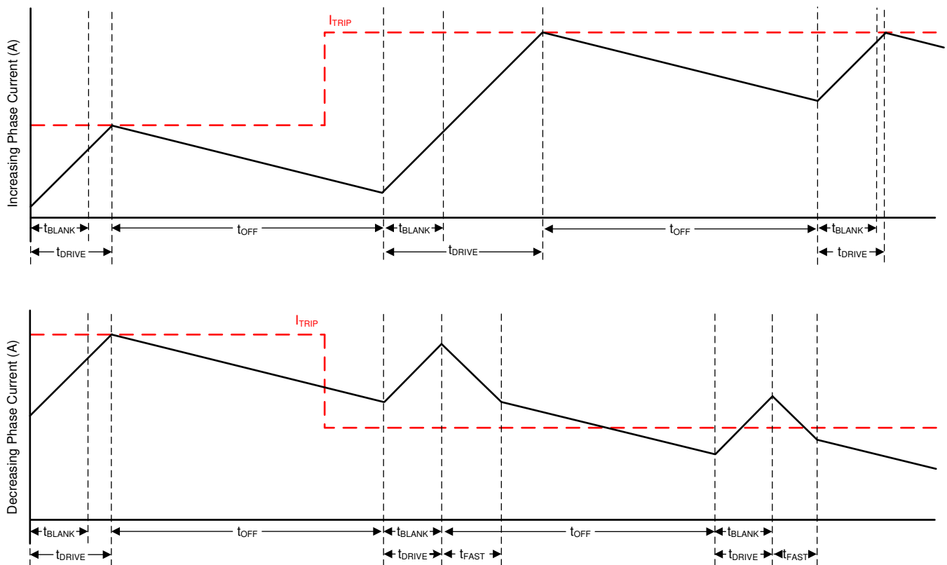
图 22. Smart tune Dynamic Decay Mode
