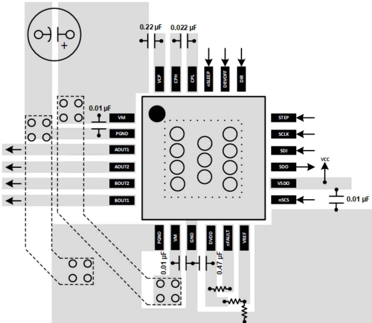
图 74. QFN Layout Recommendation
