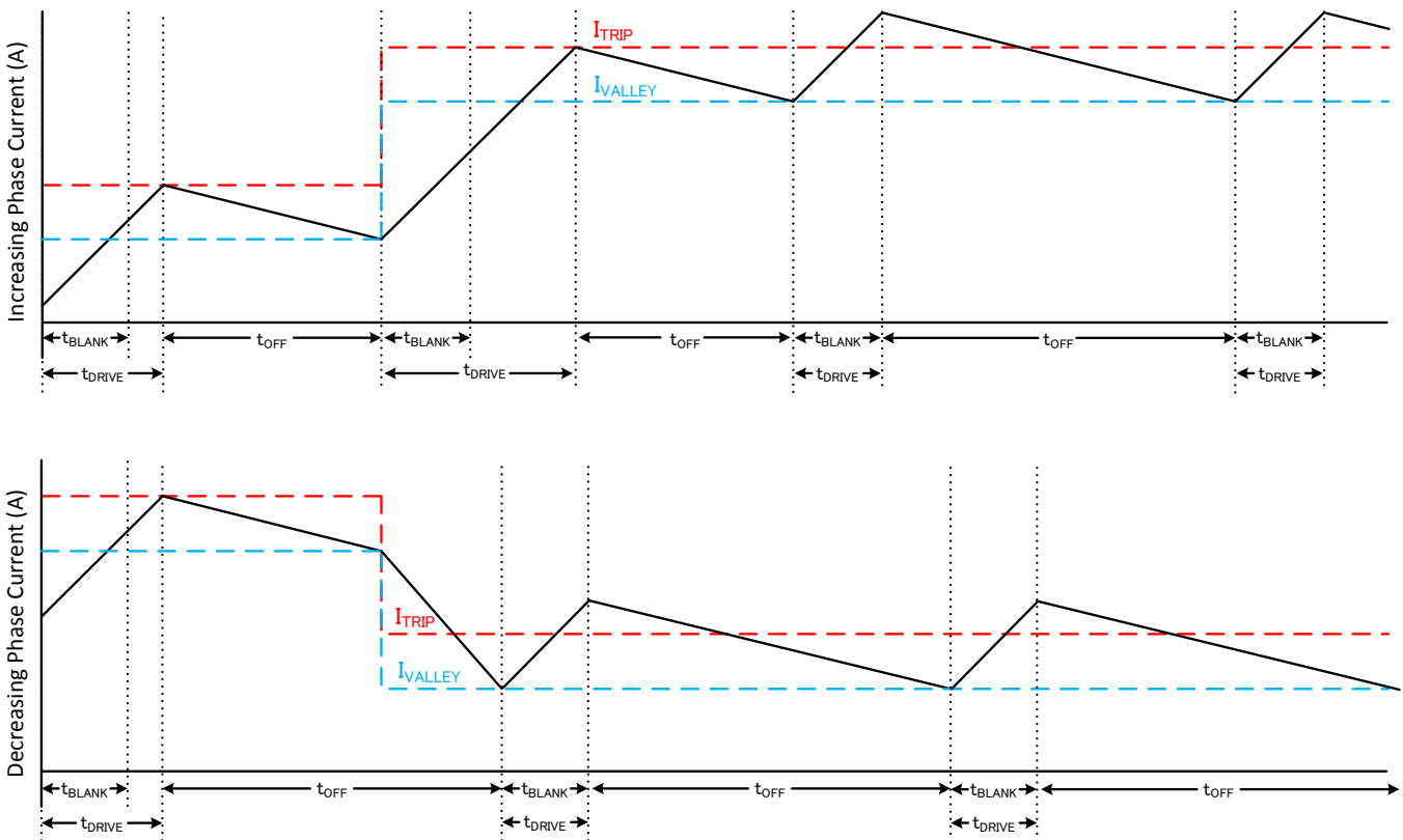
图 23. Smart tune Ripple Control Decay Mode
