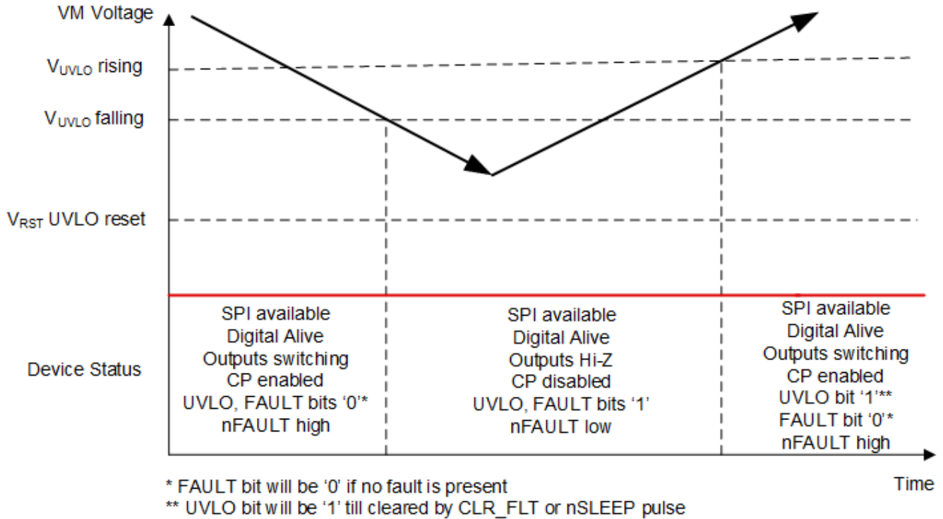
图 29. Supply Voltage Ramp Profile
