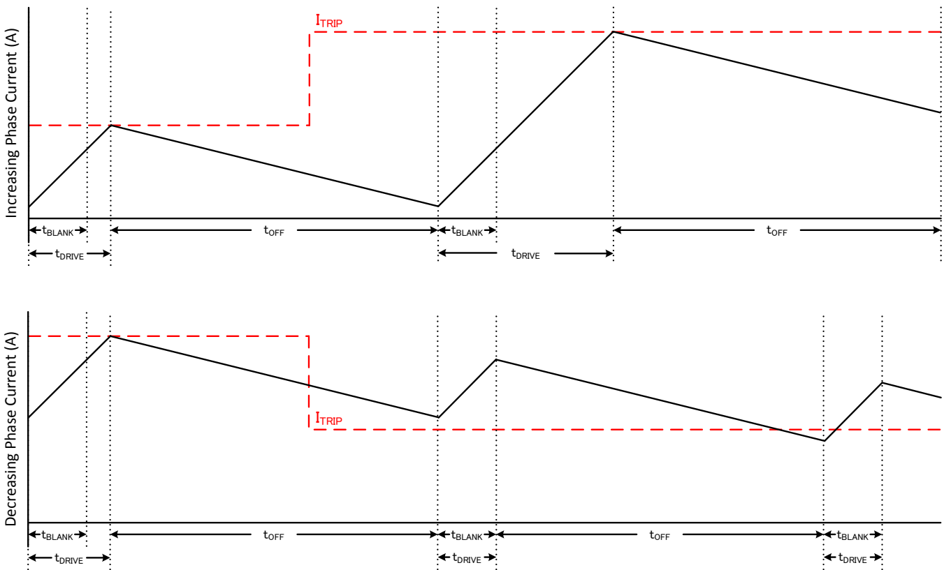
图 18. Slow/Slow Decay Mode
