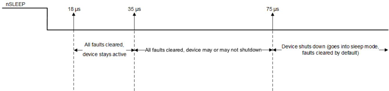
图 32. nSLEEP Reset Pulse
