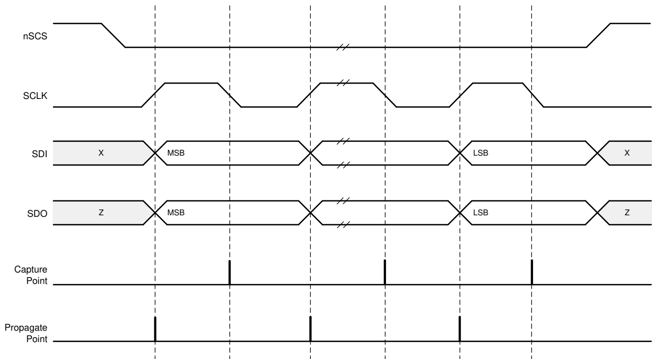
图 40. SPI Transaction
