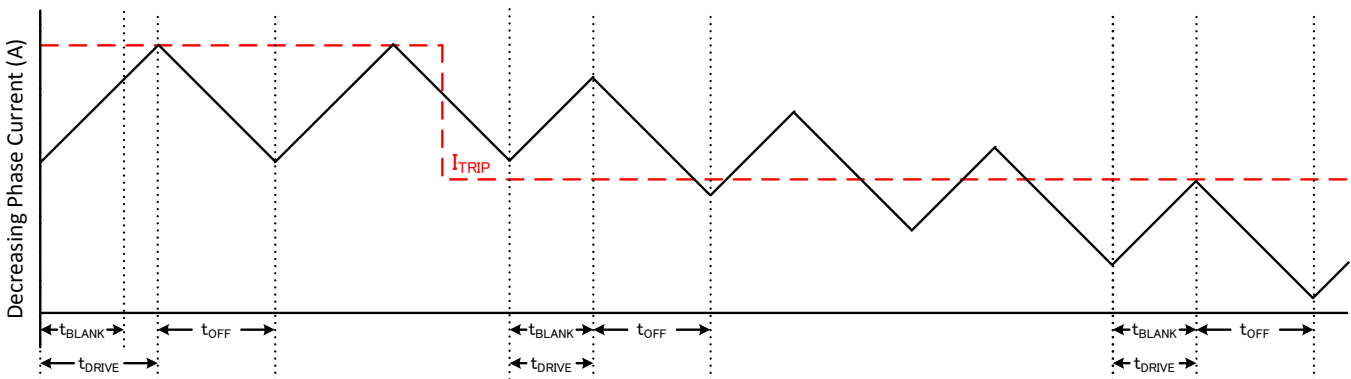
图 20. Slow/Fast Decay Mode
