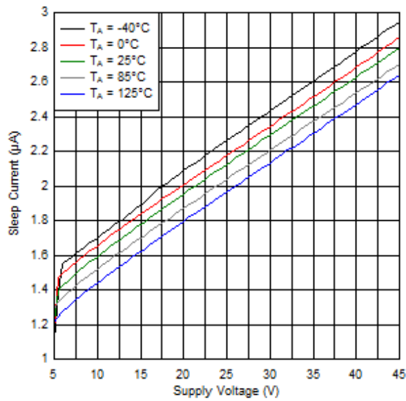
图 3. Sleep Current over VM
