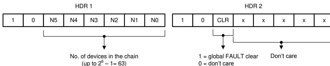
图 38. Header Bytes
