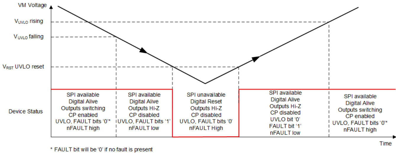
图 30. Supply Voltage Ramp Profile
