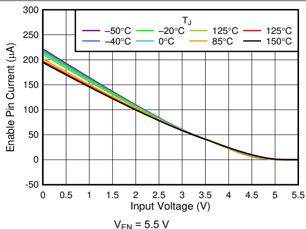
图 6-28. I_{EN} vs V_{IN}
