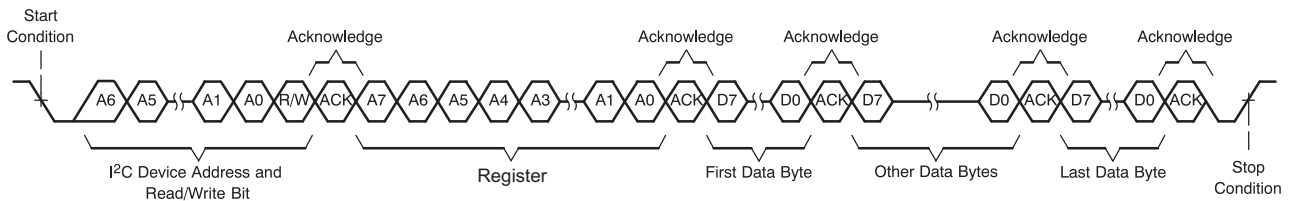
图 24. Multiple-Byte Write Transfer
