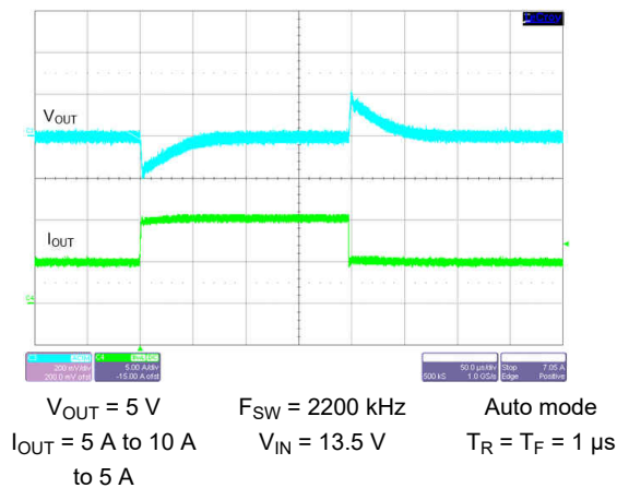
图 9-45. Load Transient
