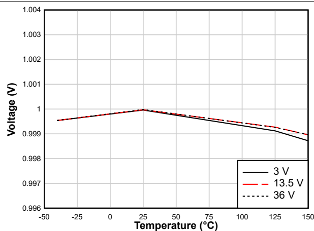
图 7-1. Feedback Voltage
