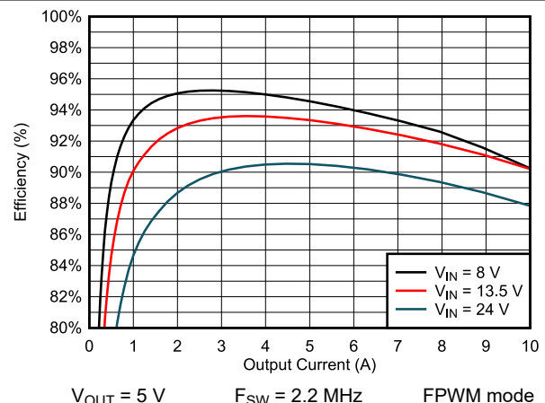
图 9-10. Efficiency
