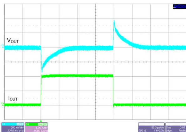
图 9-38. Load Transient
