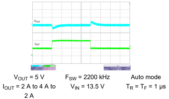
图 9-44. Load Transient
