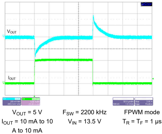
图 9-43. Load Transient
