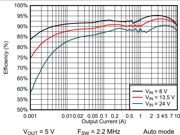
图 9-9. Efficiency
