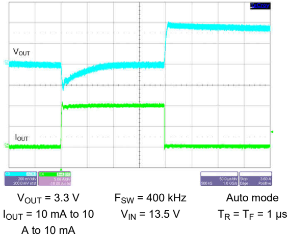
图 9-41. Load Transient
