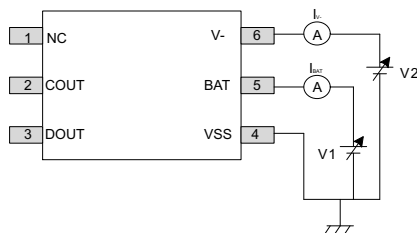
图 8-5. Test Circuit 3
