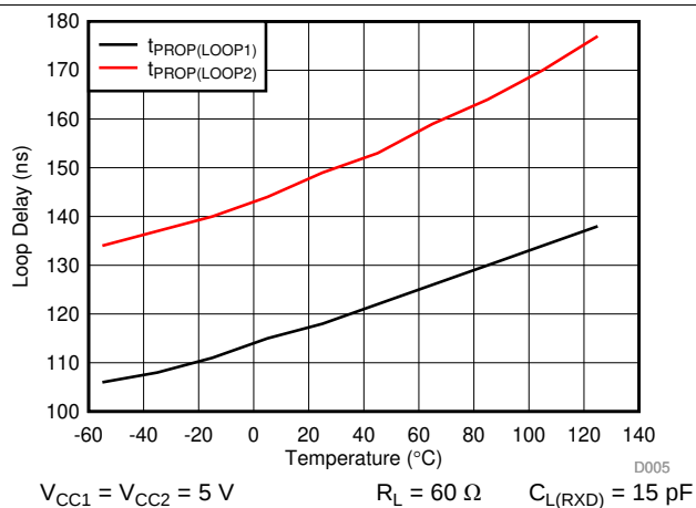
图 9. Loop Delay vs Ambient Temperature
