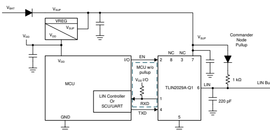
简化原理图，指挥官模式 (1)
