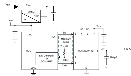
简化原理图，响应者模式 (2)
