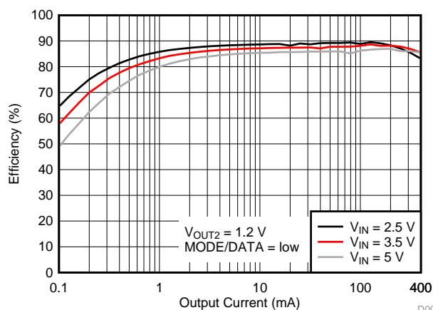
TPS62406-Q1 效率与输出电流, V_{OUT2}
