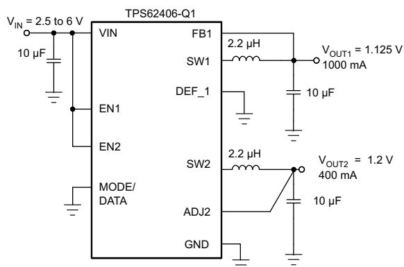
简化原理图
