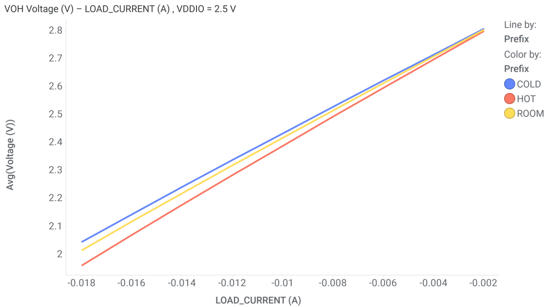
图 7-10. LED pins VOL (2.5 V)
