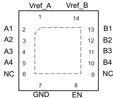
图 6-2. RGY Package 14-Pin VQFN Transparent Top View
