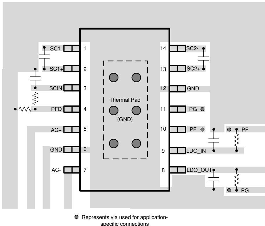
图 37. Example Layout
