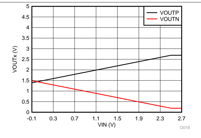
图 22. Output Voltage vs Input Voltage
