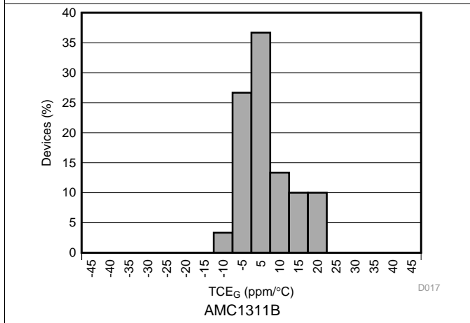
图 19. Gain Error Drift Histogram
