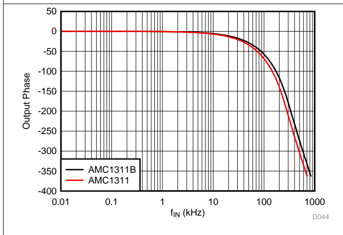
图 21. Output Phase vs Input Frequency
