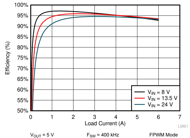
图 10-10. LM61460-Q1 Efficiency
