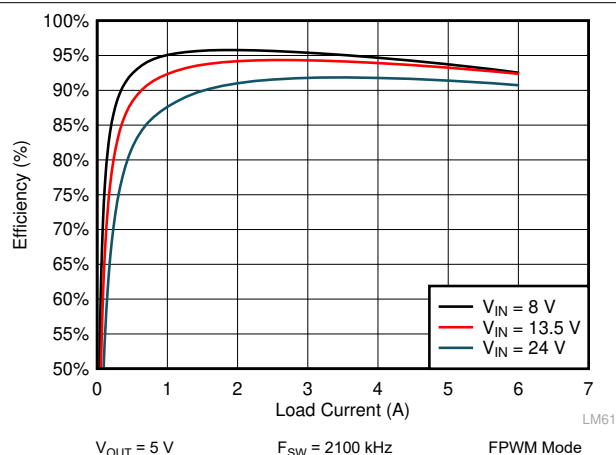
图 10-12. LM61460-Q1 Efficiency
