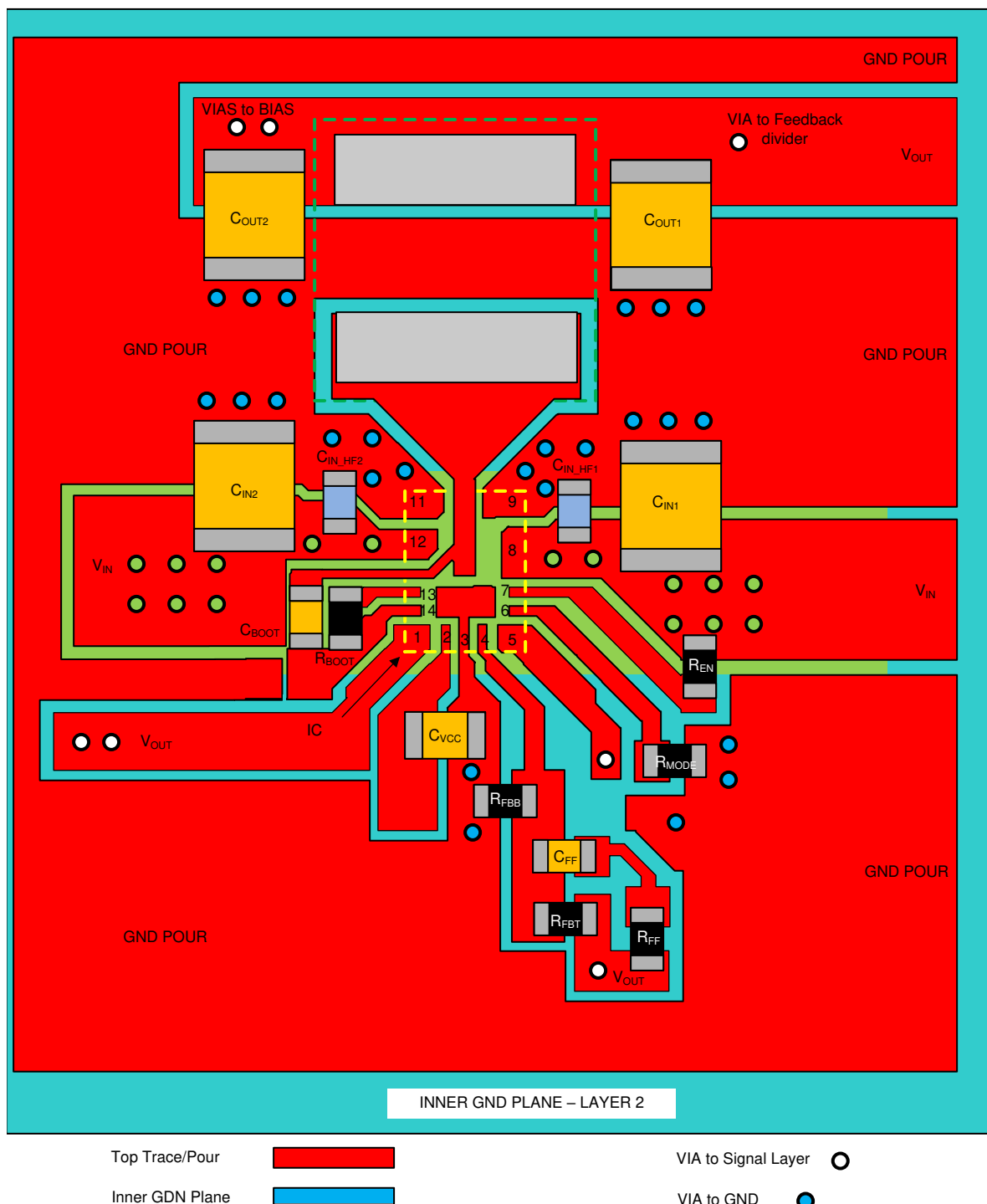
图 12-2. Layout Example
