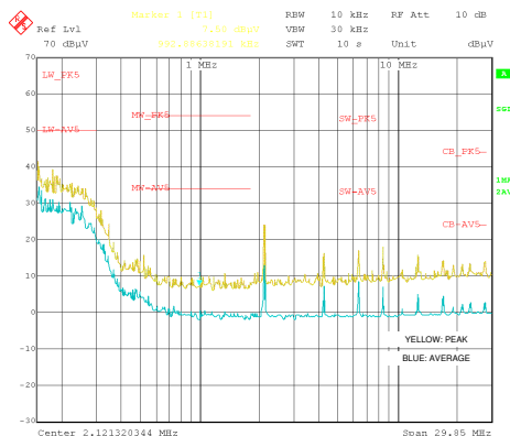
传导 EMI: V_{OUT} = 5V , I_{OUT} = 5A
