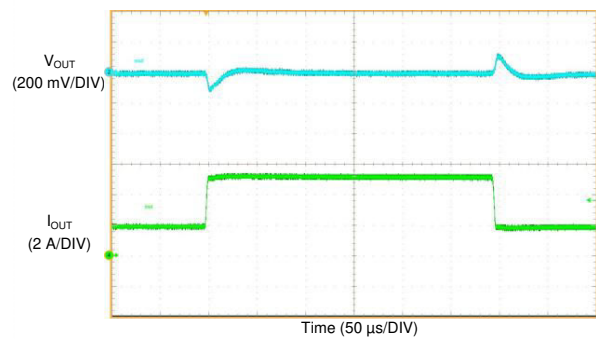
图 10-38. LM61460-Q1 Load Transient
