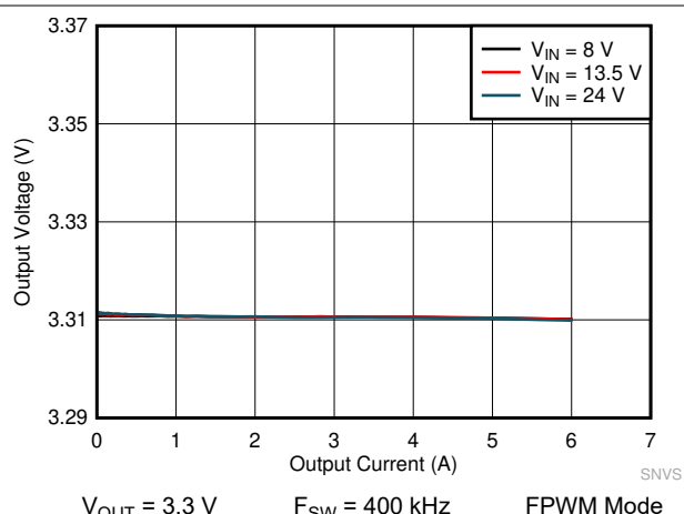
图 10-14. LM61460-Q1 Load and Line Regulation
