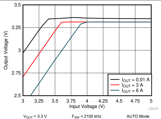
图 10-22. LM61460-Q1 Dropout Curve
