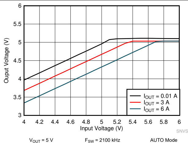
图 10-24. LM61460-Q1 Dropout Curve
