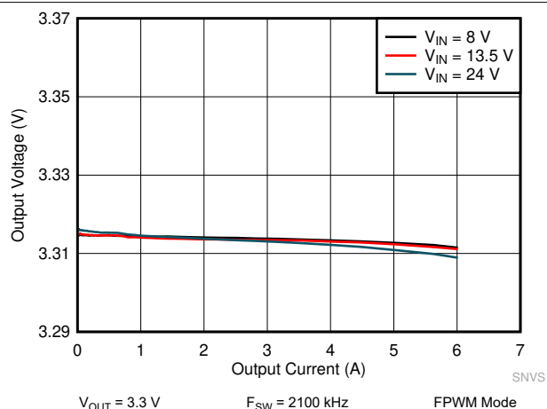
图 10-16. LM61460-Q1 Load and Line Regulation
