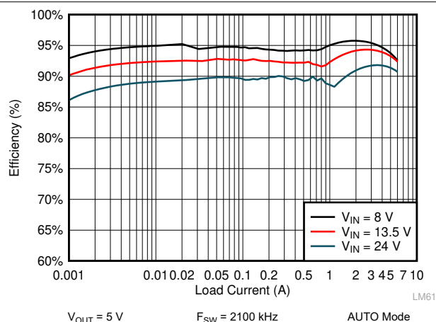
图 10-11. LM61460-Q1 Efficiency
