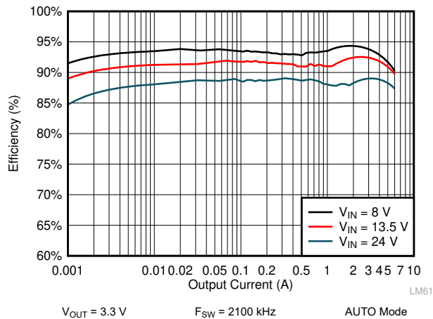
图 10-7. LM61460-Q1 Efficiency
