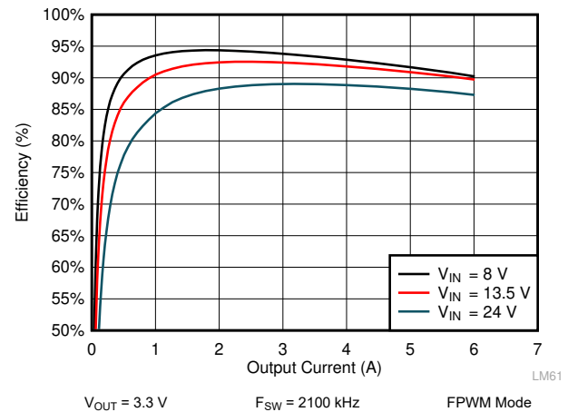
图 10-8. LM61460-Q1 Efficiency
