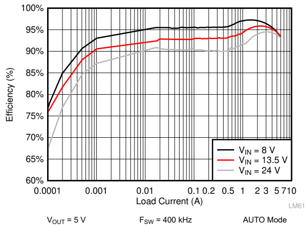
图 10-9. LM61460-Q1 Efficiency
