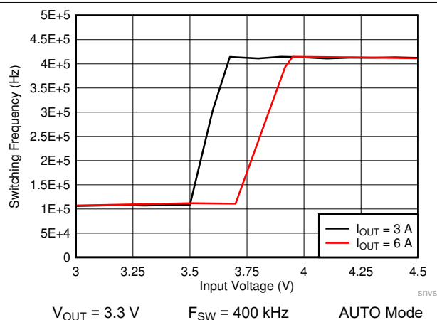
图 10-25. LM61460-Q1 Frequency Dropout
