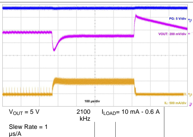
图 54. Load Transient
