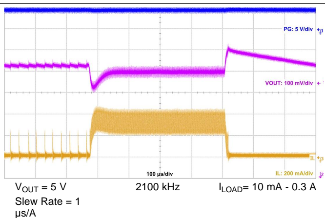
图 52. Load Transient
