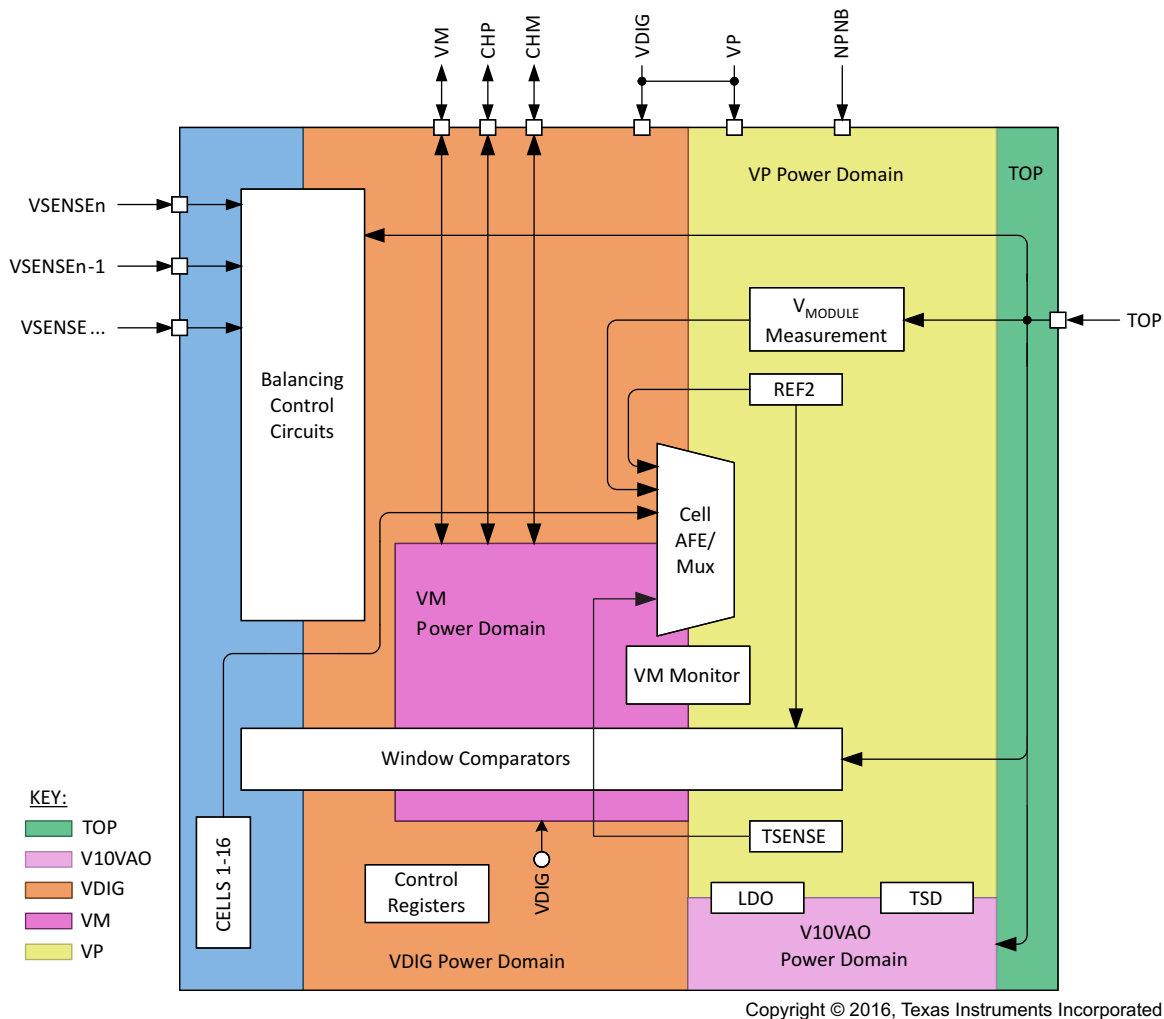
图 15. Analog Die Power Domains
