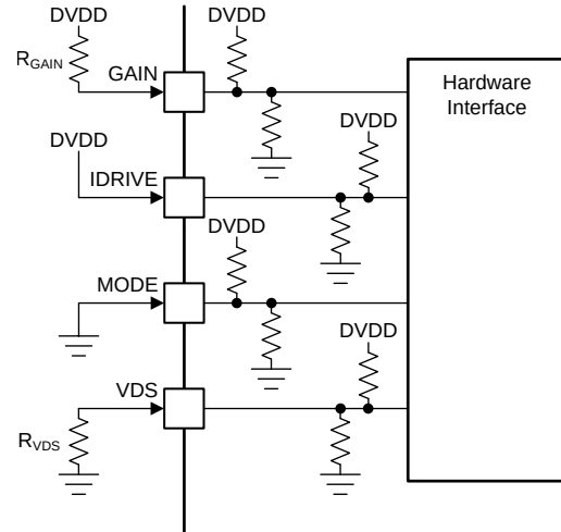
图 17. Hardware Interface
