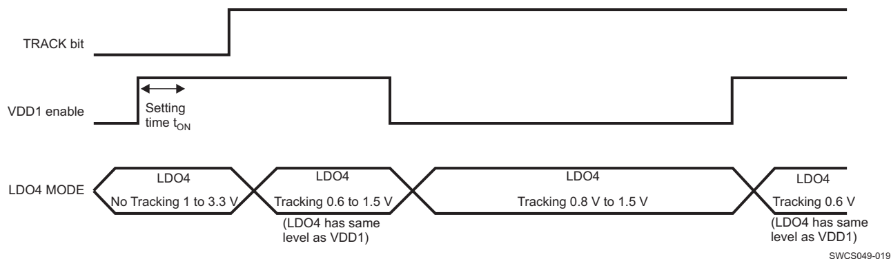
图 19. Tracking LDO
