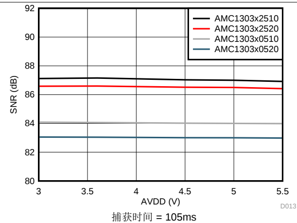
图 16. 信噪比与高侧电源电压间的关系
