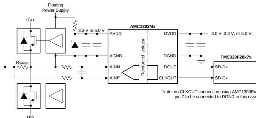
简化原理图
