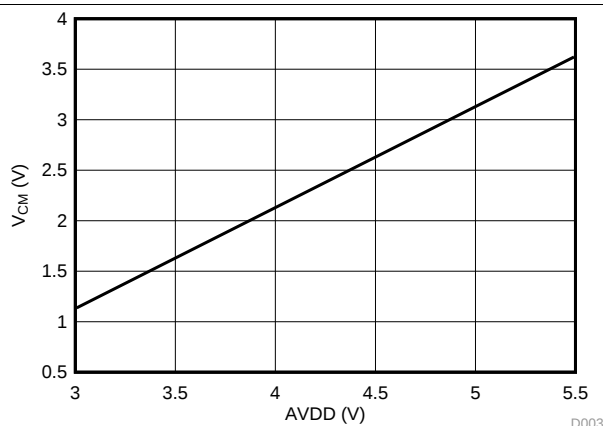
图 6. 最大工作共模输入电压与高侧电源电压间的关系
