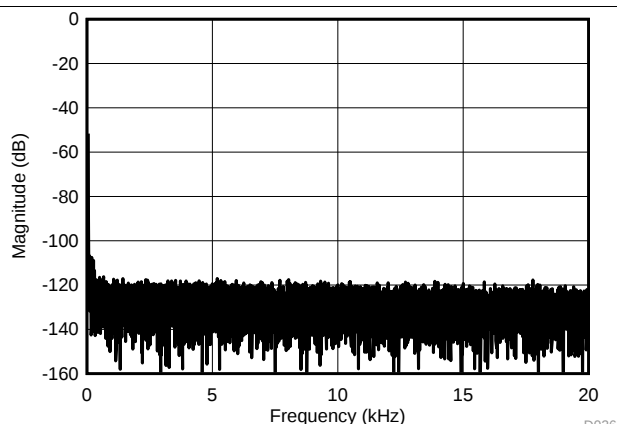
AMC1303x2520, 捕获时间 = 839ms, V_{IN} = 500\text{mV}_{PP}
