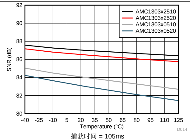
图 17. 信噪比与温度间的关系
