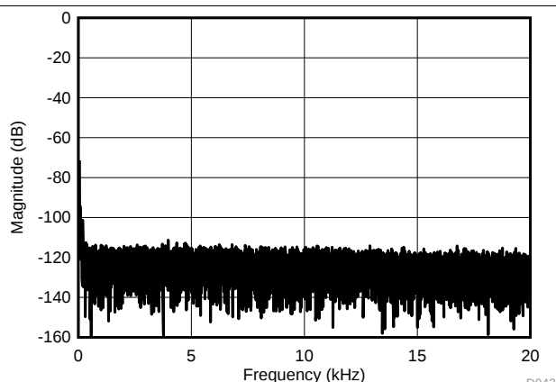
AMC1303x0520, 捕获时间 = 839ms, V_{IN} = 100\text{mV}_{PP}
