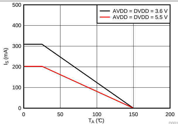
图 3. 安全限制电流的热降额曲线（符合 VDE）
