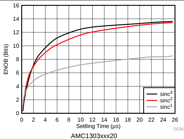
图 53. 测得的有效位数与建立时间间的关系
