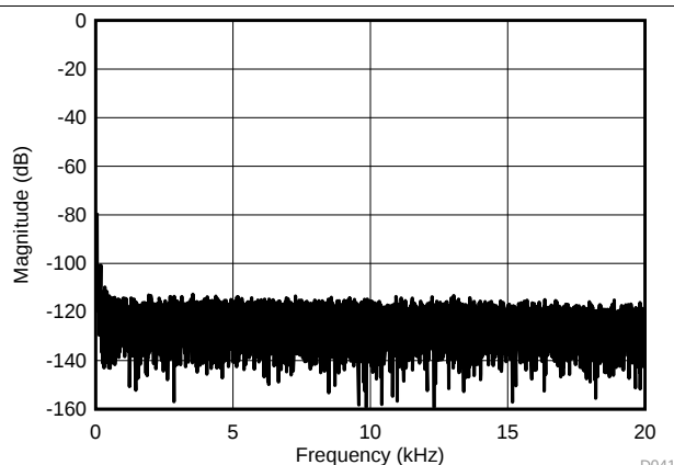
AMC1303x0510, 捕获时间 = 839ms, V_{IN} = 100\text{mV}_{PP}
