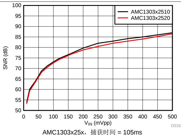
图 19. 信噪比与输入信号幅度间的关系
