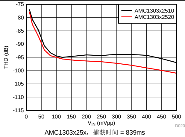
图 24. 总谐波失真与输入信号幅度间的关系
