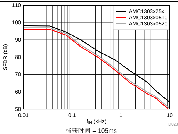
图 28. 无杂散动态范围与输入信号频率间的关系
