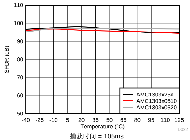
图 27. 无杂散动态范围与温度间的关系
