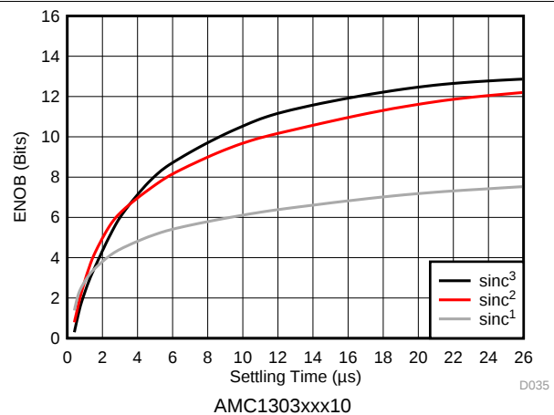
图 54. 测得的有效位数与建立时间间的关系
