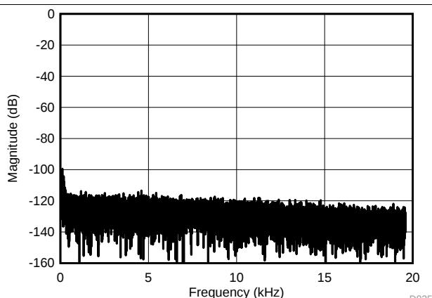
AMC1303x2510, 捕获时间 = 839ms, V_{IN} = 500\text{mV}_{PP}
