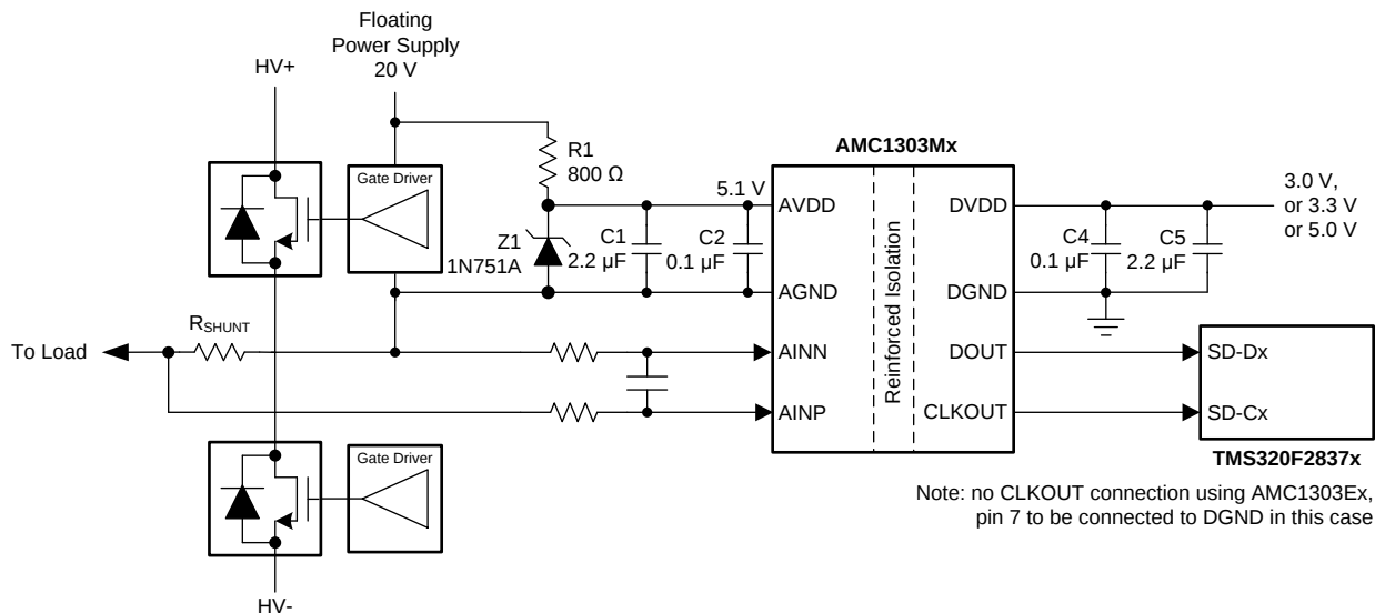
图 57. 对 AMC1303 去耦
