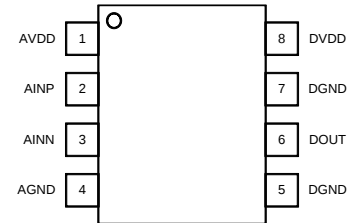
AMC1303Ex: DWV 封装 8 引脚 SOIC 俯视图
