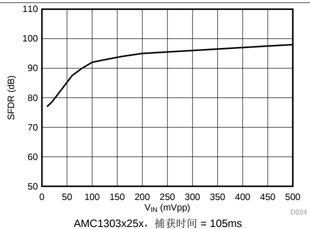
图 29. 无杂散动态范围与输入信号幅度间的关系
