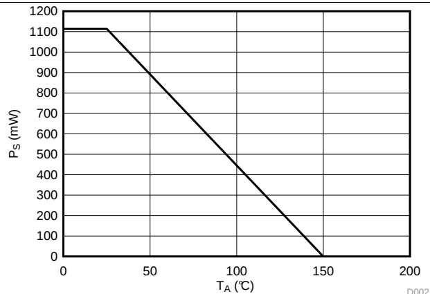
图 4. 安全限制功耗的热降额曲线（符合 VDE）
