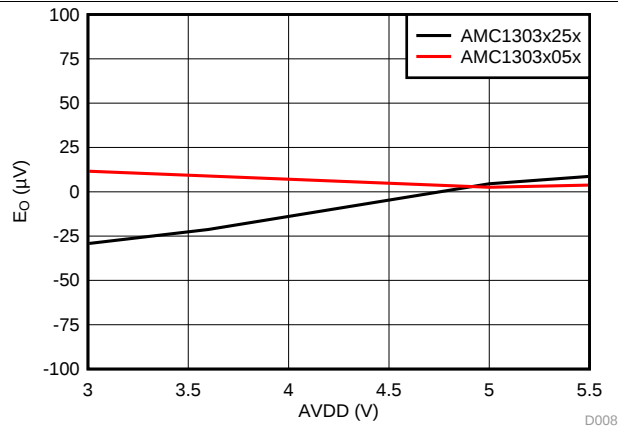
图 12. 失调误差与高侧电源电压间的关系
