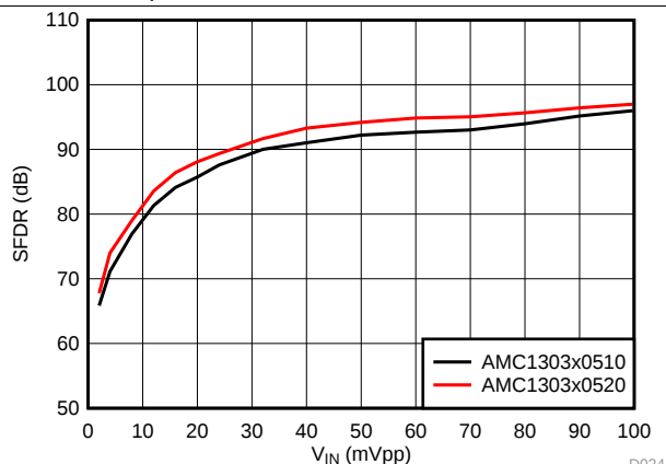
AMC1303x05x, 捕获时间 = 105ms
