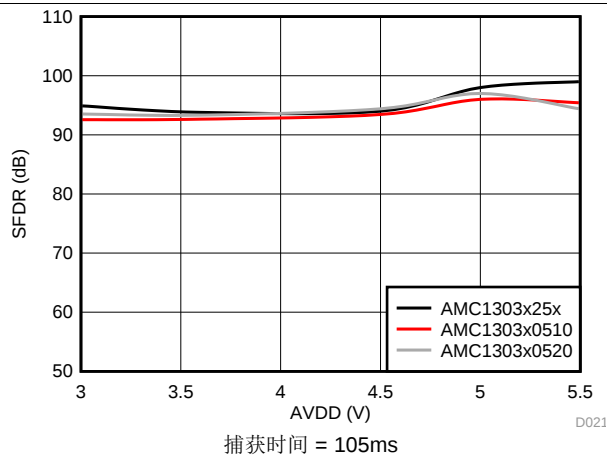
图 26. 无杂散动态范围与高侧电源电压间的关系
