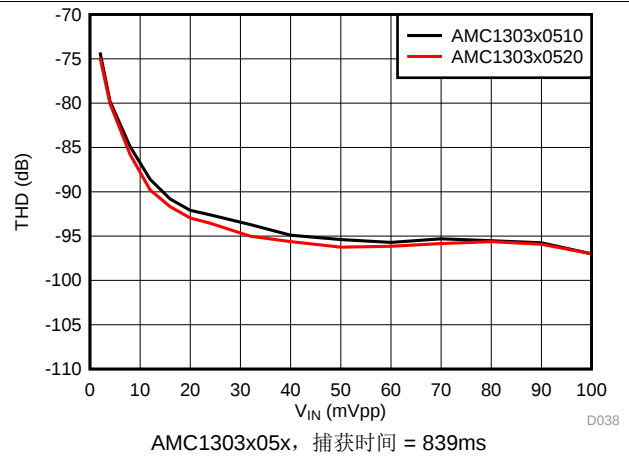
图 25. 总谐波失真与输入信号幅度间的关系
