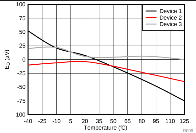
图 13. 失调误差与温度间的关系
