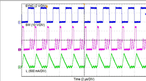
图 7-7. Synchronizing in DCM
