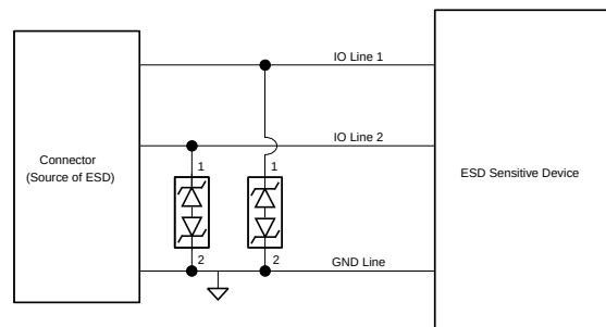
应用电路原理图
