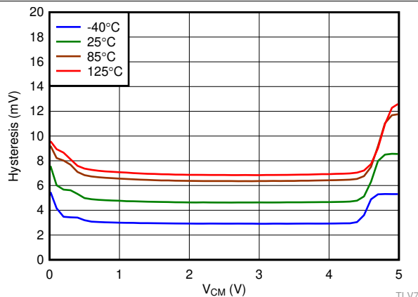
图 11. Hysteresis vs. V_{CM}
