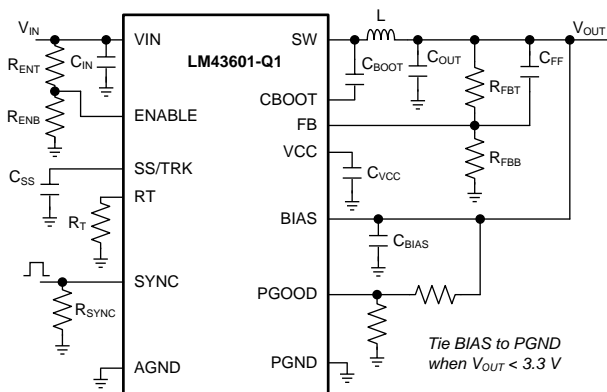
简化原理图
