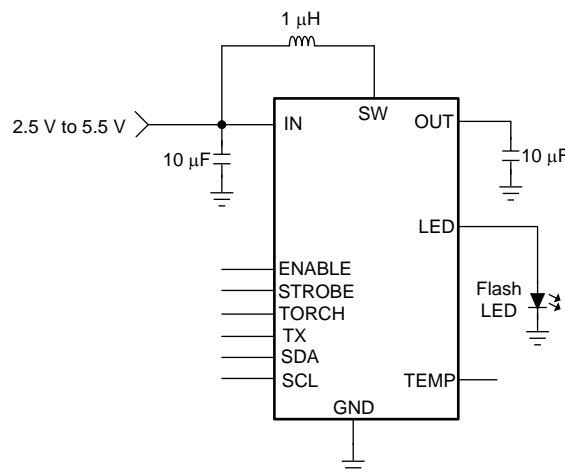
典型应用电路
