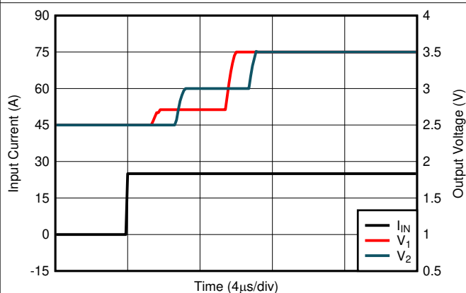
图 7-9. Voltage Output Step, Rising
