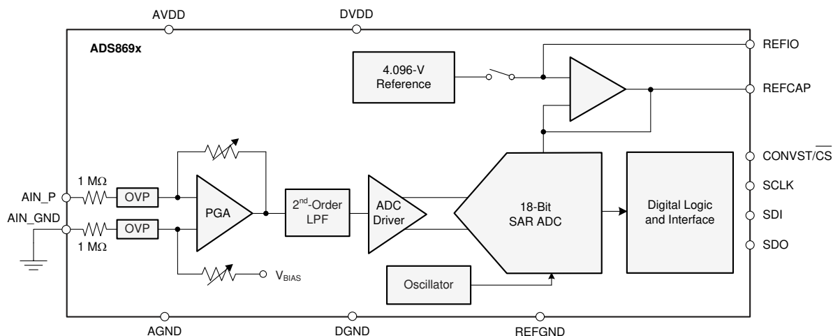
方框图
