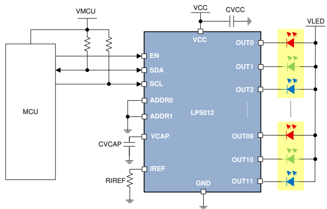
简化原理图
