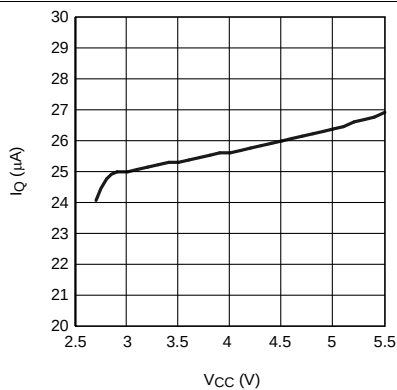
图 3. 静态电流与 VCC 间的关系
