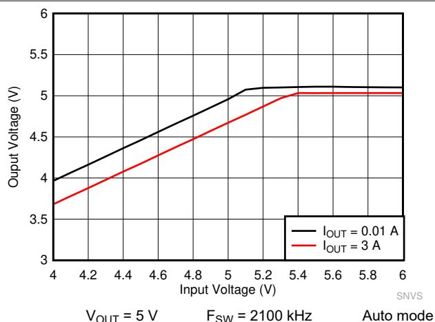
图 9-23. LM61430-Q1 Dropout Curve
