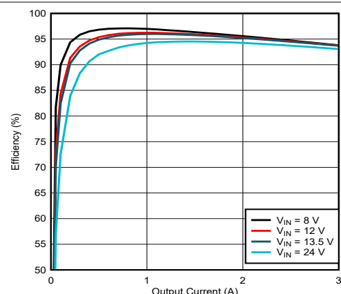
图 9-7. LM61430-Q1 Efficiency
