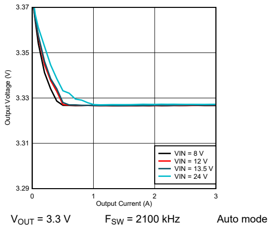
图 9-14. LM61430-Q1 Load and Line Regulation
