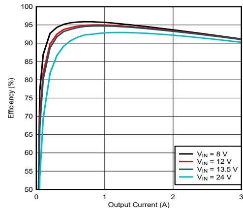
图 9-5. LM61430-Q1 Efficiency
