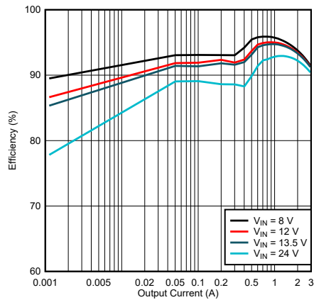
图 9-4. LM61430-Q1 Efficiency
