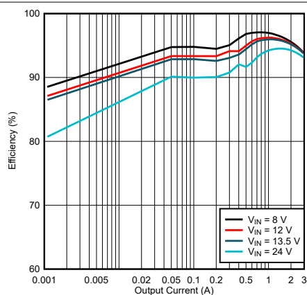
图 9-6. LM61430-Q1 Efficiency
