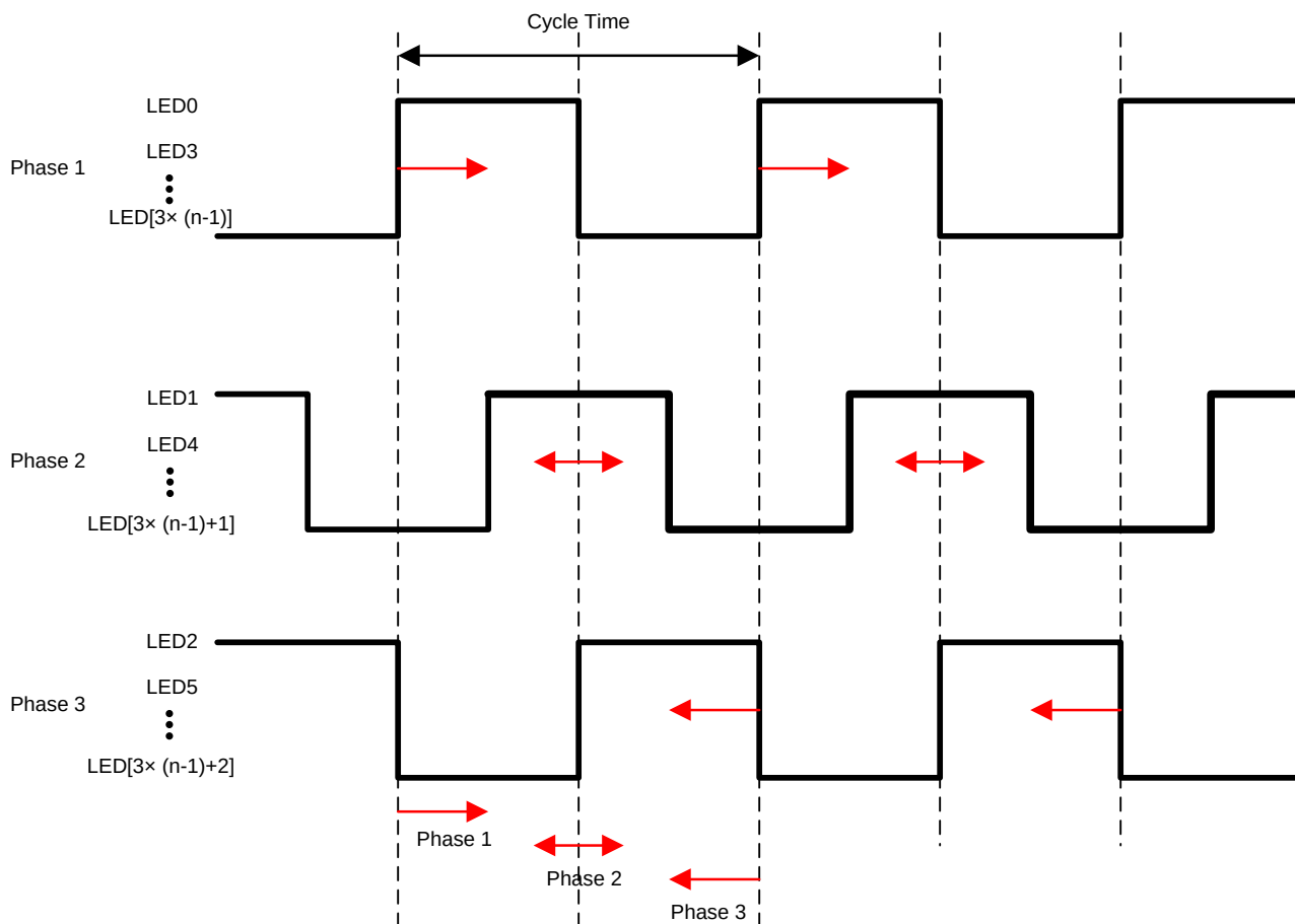
图 12. PWM Phase-Shifting
