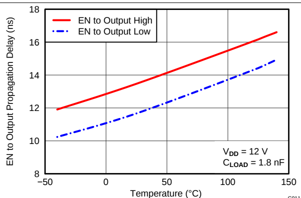
图 14. En to Output Propagation Delay vs Temperature
