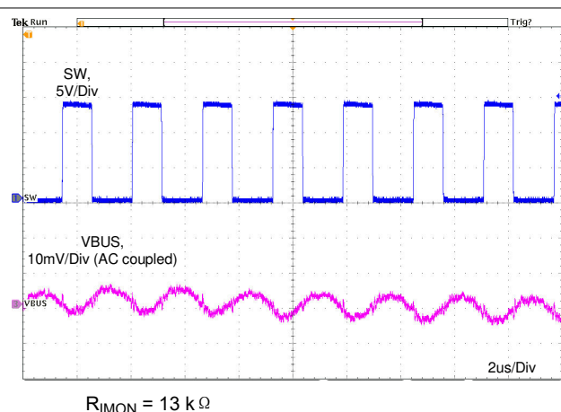
图 11-13. 3.5-A Output Ripple
