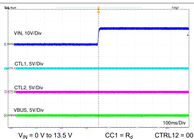
图 11-43. Client mode Startup
