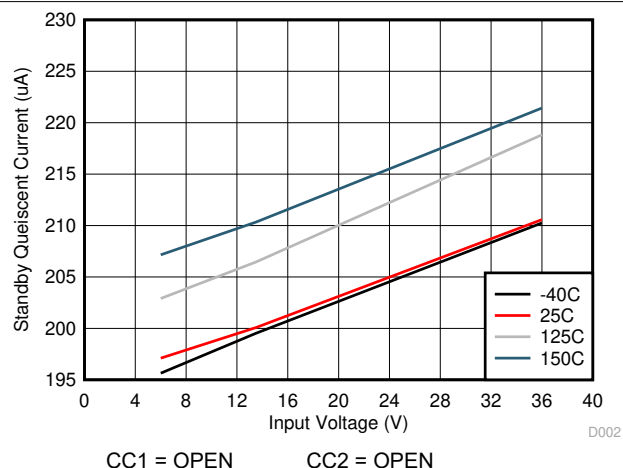
图 8-2. Standby Quiescent Current
