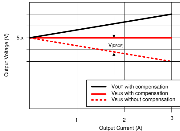
图 10-25. Voltage Drop
