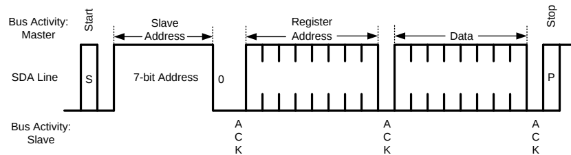
Figure 25. Write Byte
