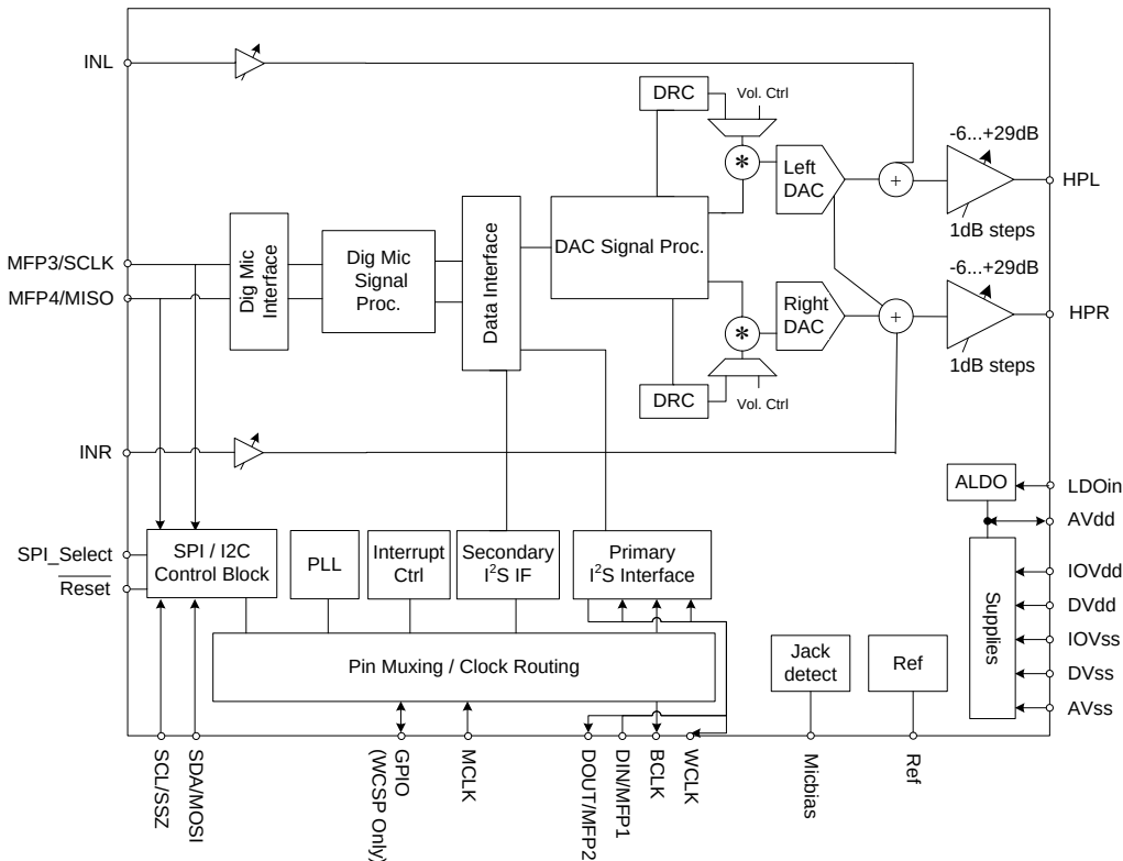
简化方框图
