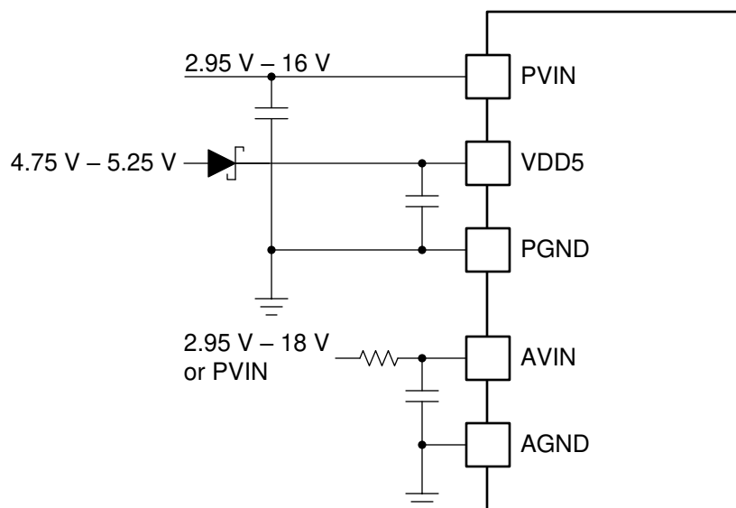
图 7-4. TPS546D24A Separate PVIN, AVIN, and VDD5 Connections
