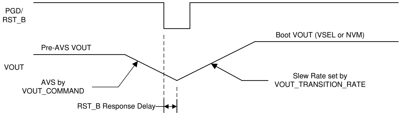
图 7-7. TPS546D24A Output Voltage Reset
