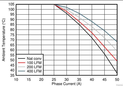
图 6-3. TPS546D24A Safe Operating Area
