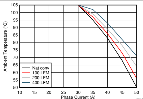
图 6-2. TPS546D24A Safe Operating Area
