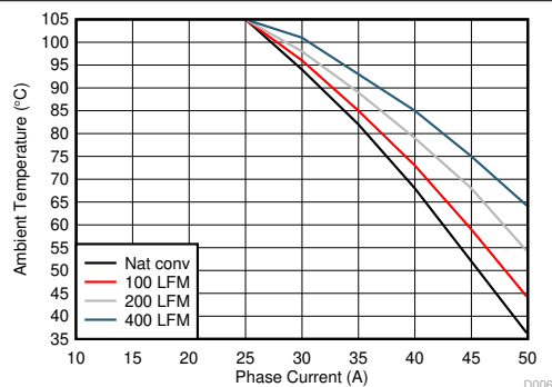
图 6-4. TPS546D24A Safe Operating Area
