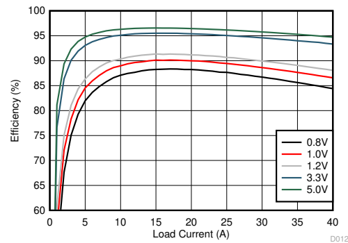
图 6-10. TPS546D24A Efficiency vs Output Current
