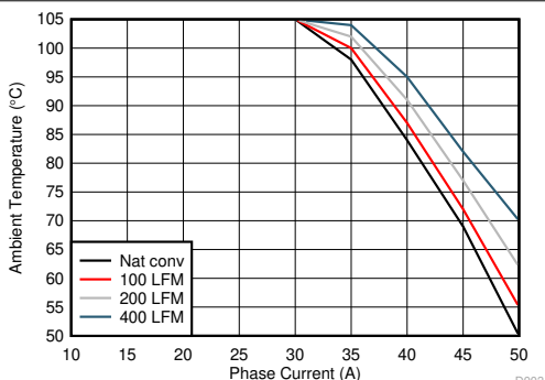
图 6-1. TPS546D24A Safe Operating Area
