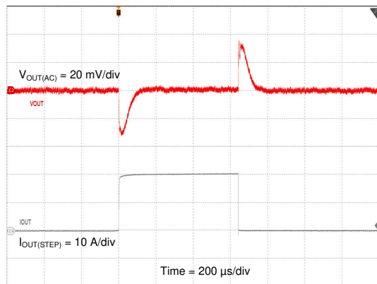
图 8-14. Load Regulation
