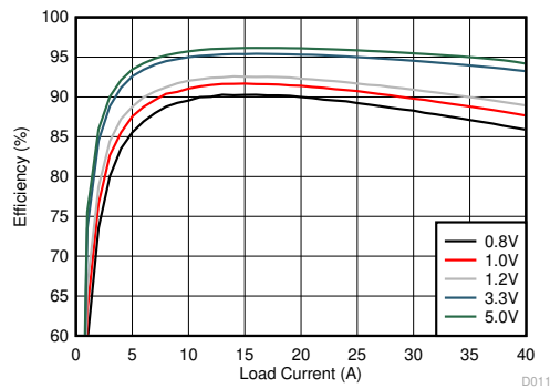
图 6-9. TPS546D24A Efficiency vs Output Current
