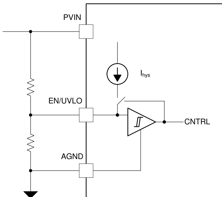
图 7-5. TPS546D24A UVLO Voltage Divider
