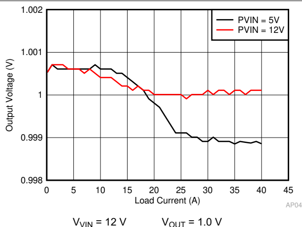
图 8-3. Load Regulation
