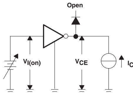
图 14. V_{I(on)} 测试电路
