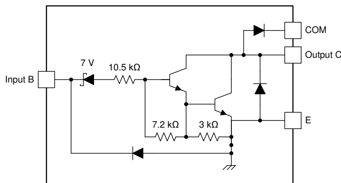
图 19. ULN2002A 方框图
