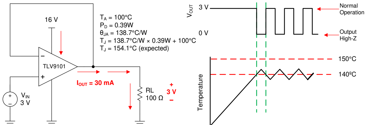
图 7-3. Thermal Protection
