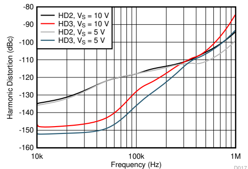
谐波失真与频率间的关系
