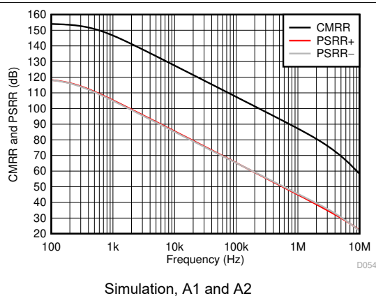
图 6-4. CMRR and PSRR vs Frequency
