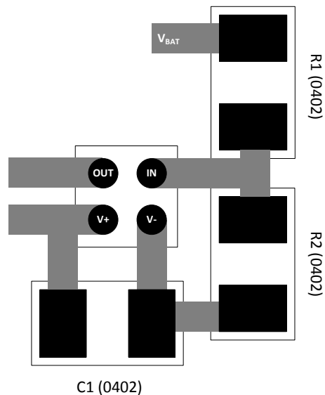
图 47. Layout Example
