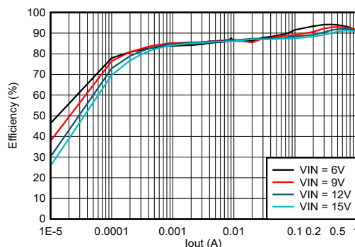
效率与输出电流间的关系 (频率为 2.5MHz 时 V_{\text{OUT}} = 3.3\text{V} , 自动 PFM/PWM)
