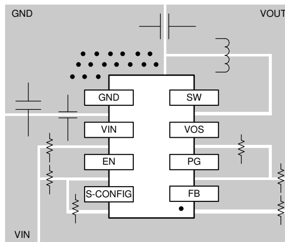
图 11-1. TPS629210-Q1 Layout
