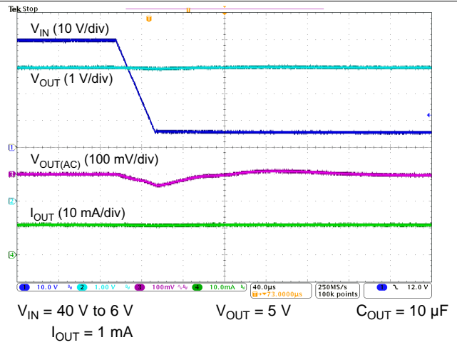
图 16. Line Transient
