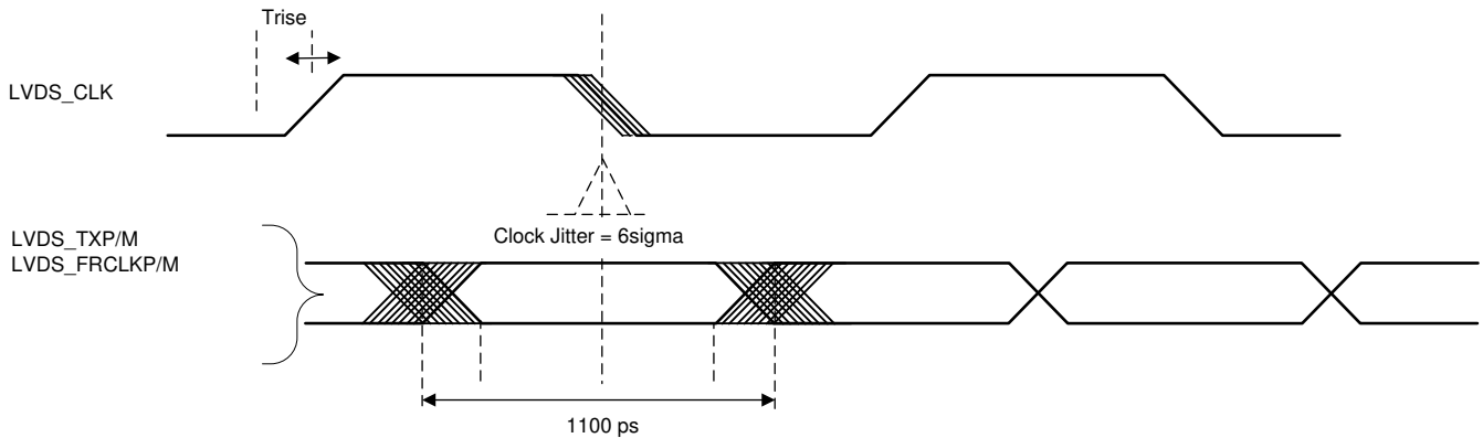
Figure 8-9. Timing Parameters
