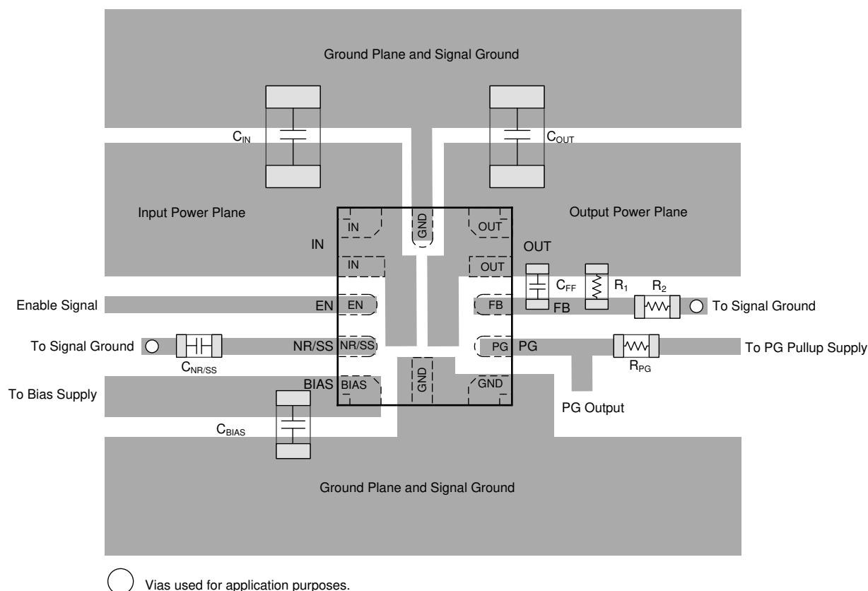
图 55. Example Layout
