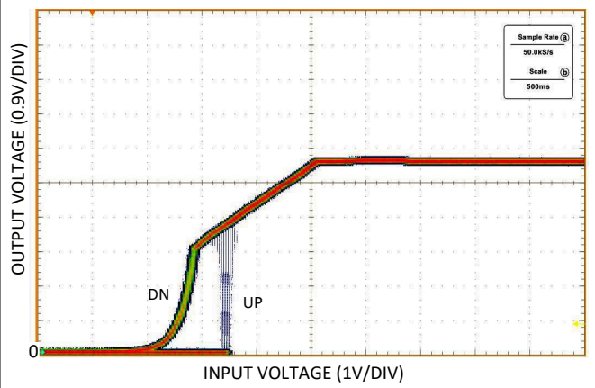
图 7-2. UVLO Thresholds
