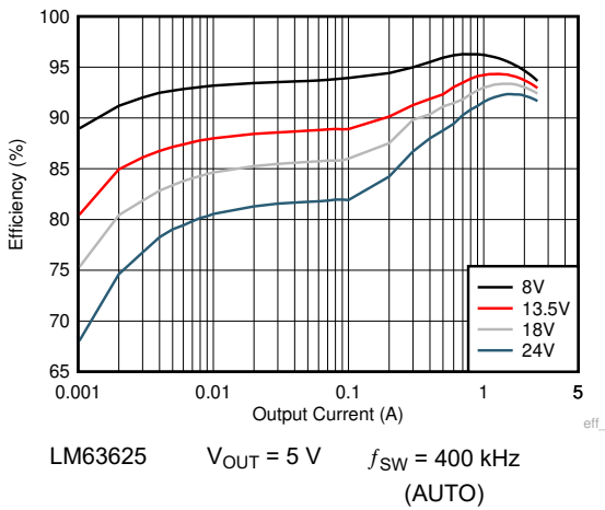
图 9-8. Efficiency
