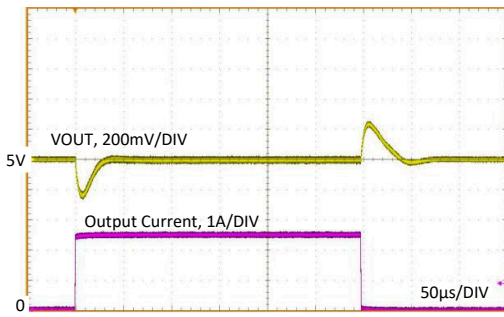
图 9-26. Load Transient
