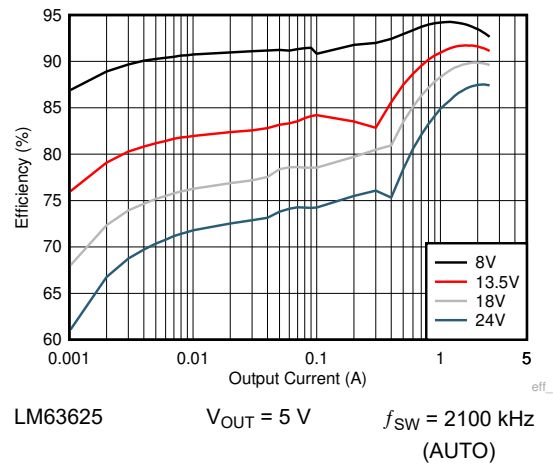
图 9-9. Efficiency
