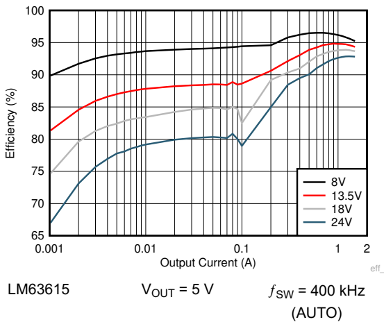
图 9-10. Efficiency
