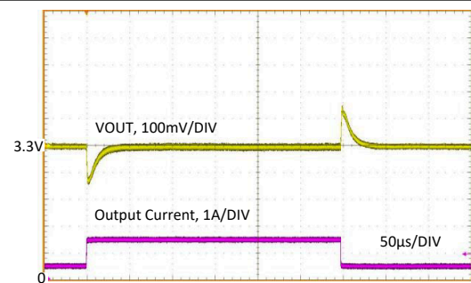
图 9-29. Load Transient
