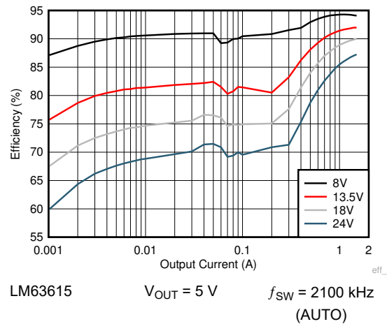
图 9-11. Efficiency
